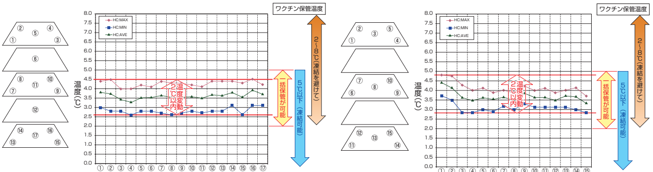
FMS-174GS 設定温度: HCモード 3℃ 周囲温度: 30℃ 周囲湿度: 60%
