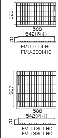
棚網寸法 (mm)
